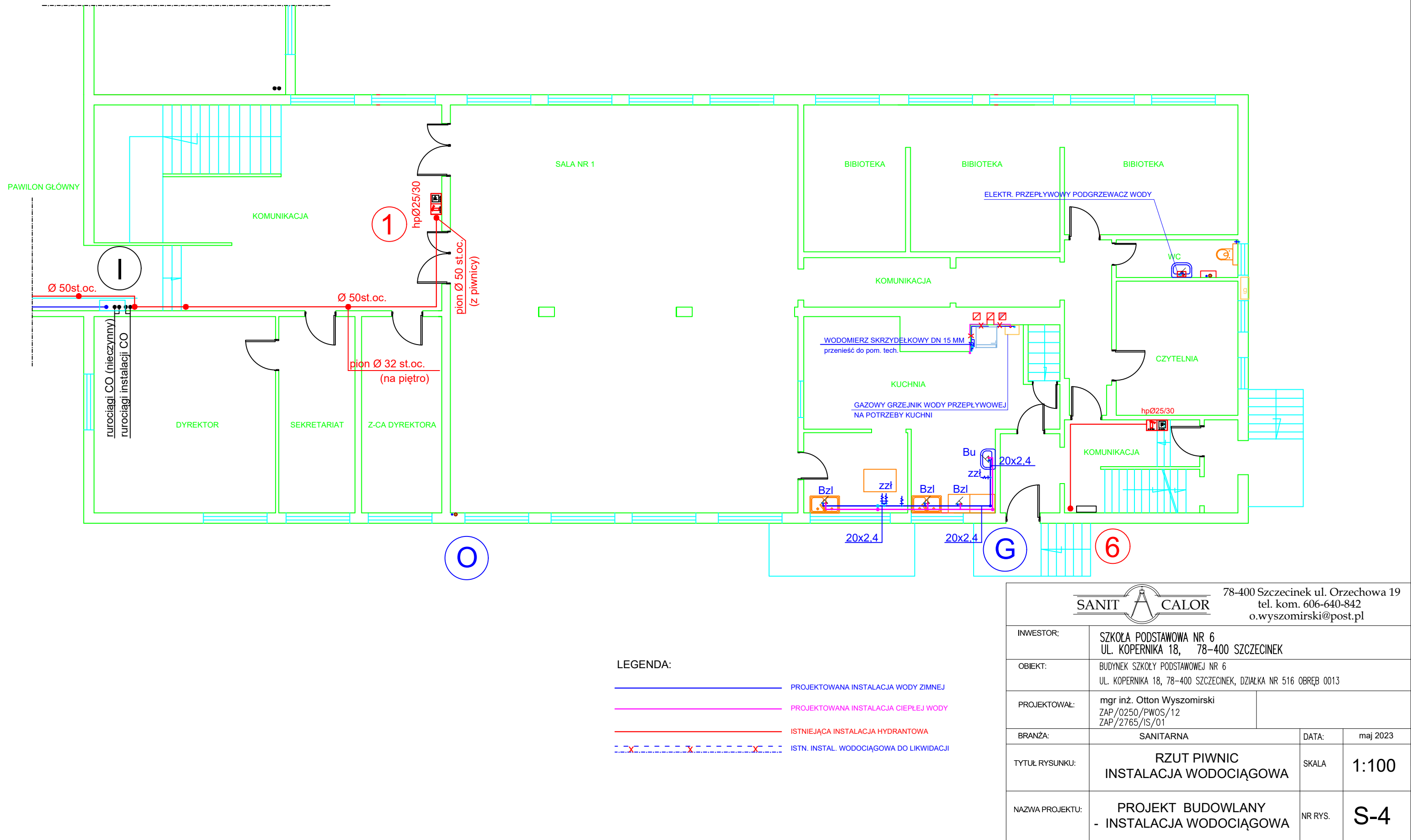
RZUT PARTERU 1:100
