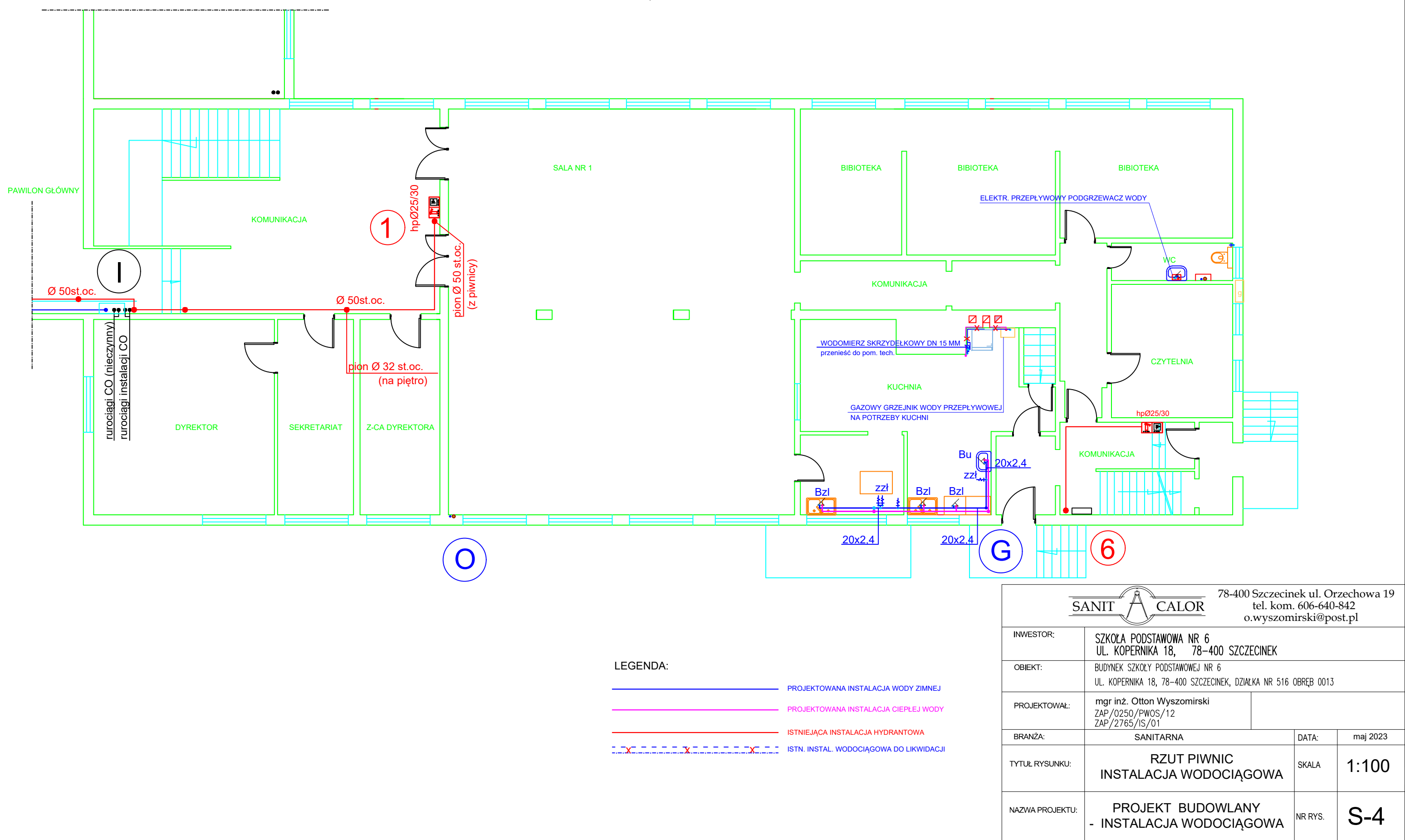
RZUT PARTERU 1:100
