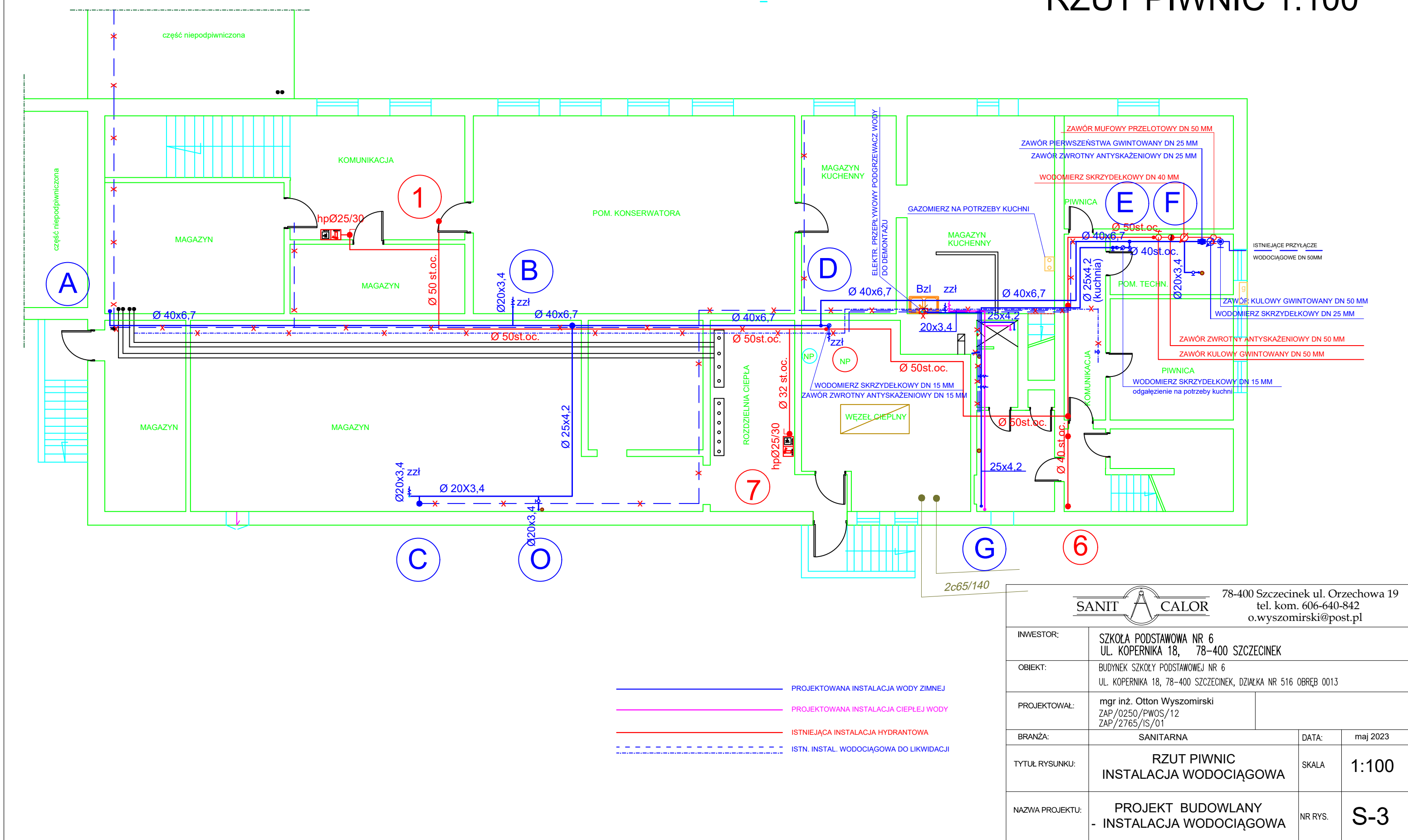
RZUT PIWNIC 1:100
